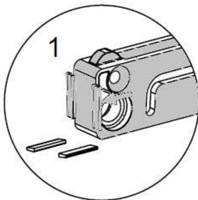
CASSER LES LANGUETTES
