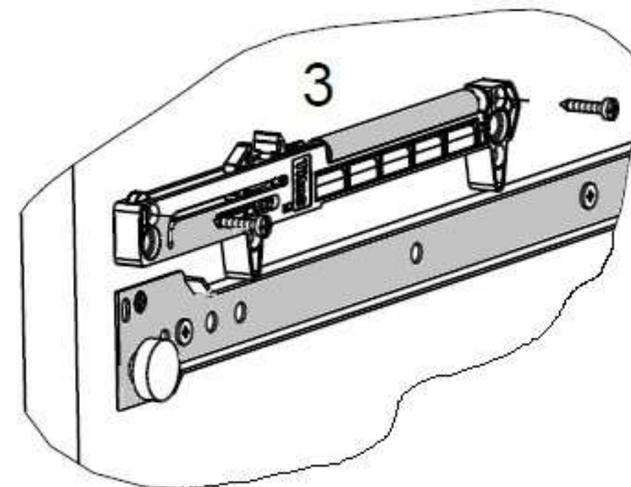
VISSER L'AMORTISSEUR A L'AIDE DES VIS
