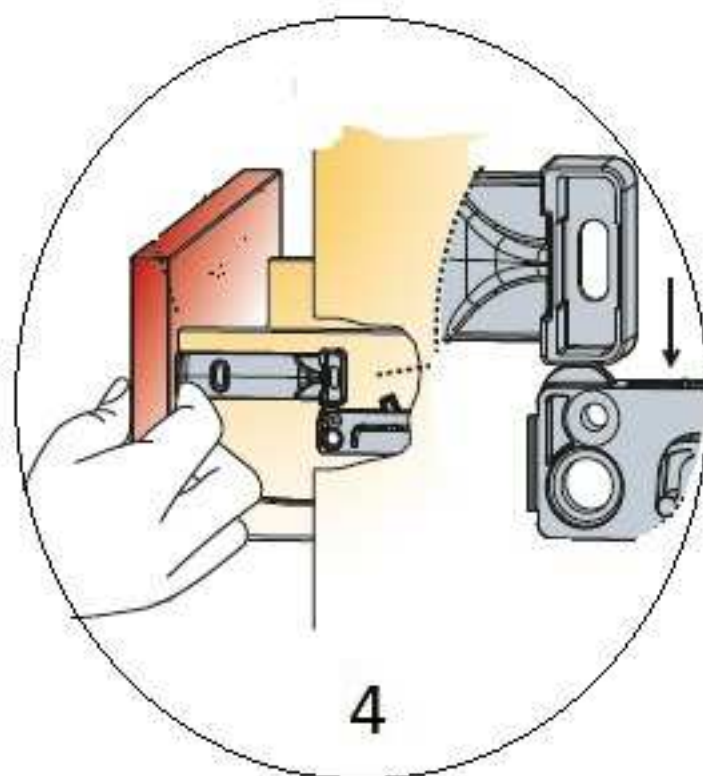
POSITIONNER L'ARRET SUR LE TIROIR
